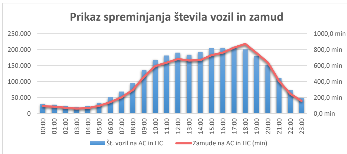
Graf 3: Prikaz spreminjanja števila vozil in zamud na omrežju (7.9.2025)
